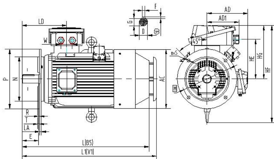
图 13 YE5 160~280 结构示意图
