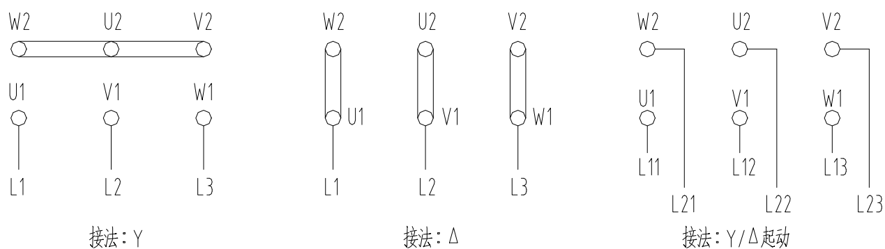
图 2 接线指示图
