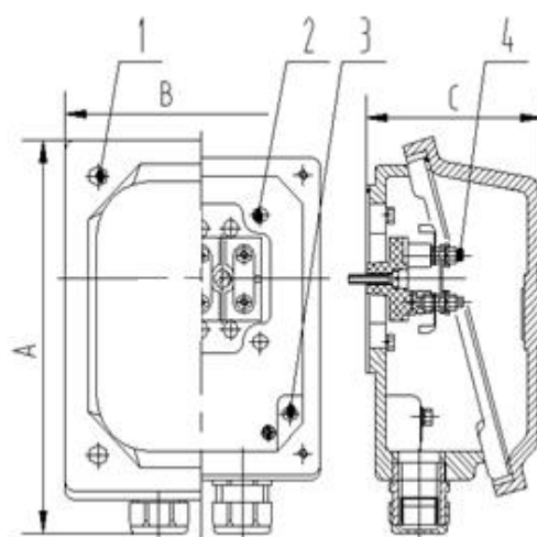
图 16 YE5 132 示意图
