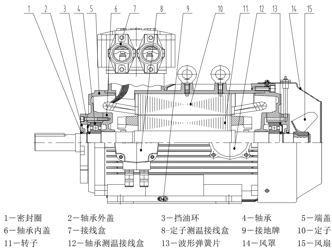
图 5 YE5 315~355 结构剖面示意图
