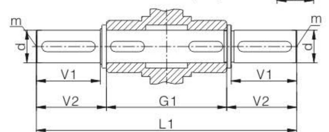
双向输出轴(SZ)
