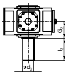
V2SV 实心轴
