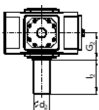
V4SV 实心轴
