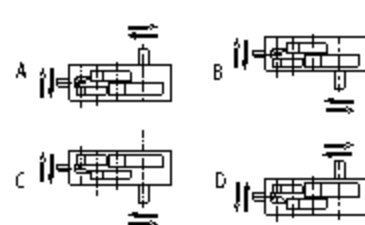
布置形式
