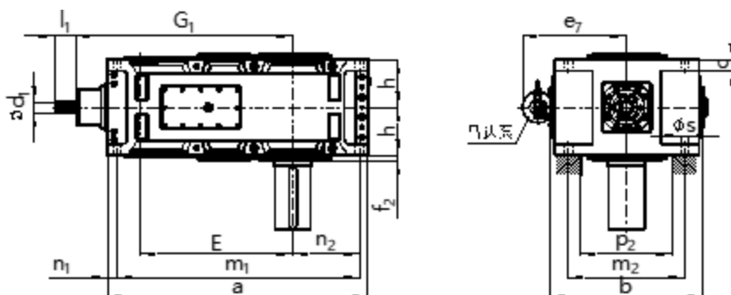
V4HV 空心轴
