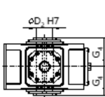
V4HV 空心轴
